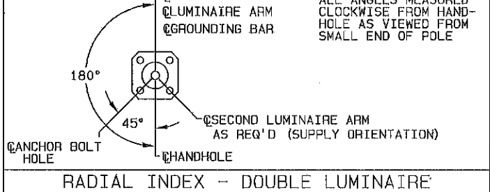
RADIAL INDEX - DOUBLE LUMINAIRE
