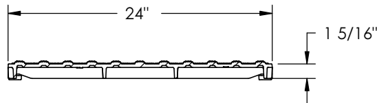
SECTION A-A
