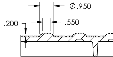
SECTION D-D SCALE 1 : 4
